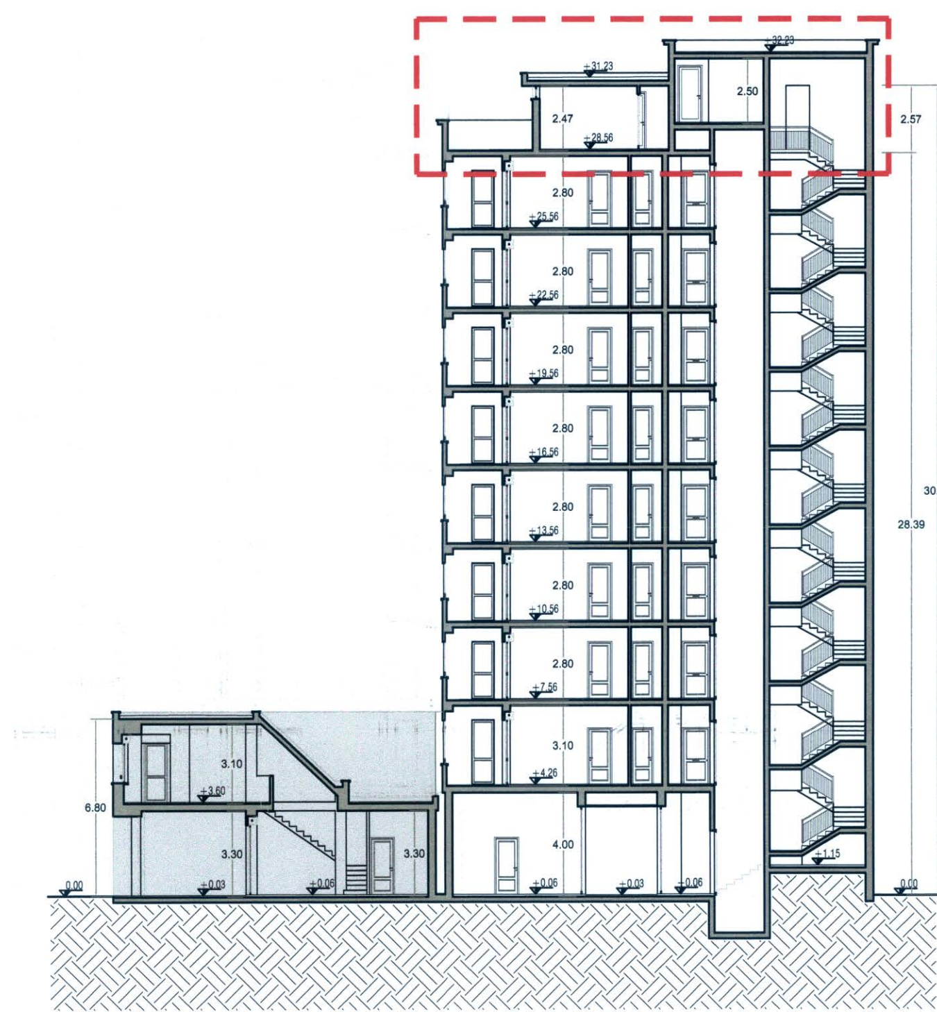
Sezione Y-Y' scala 1:200
