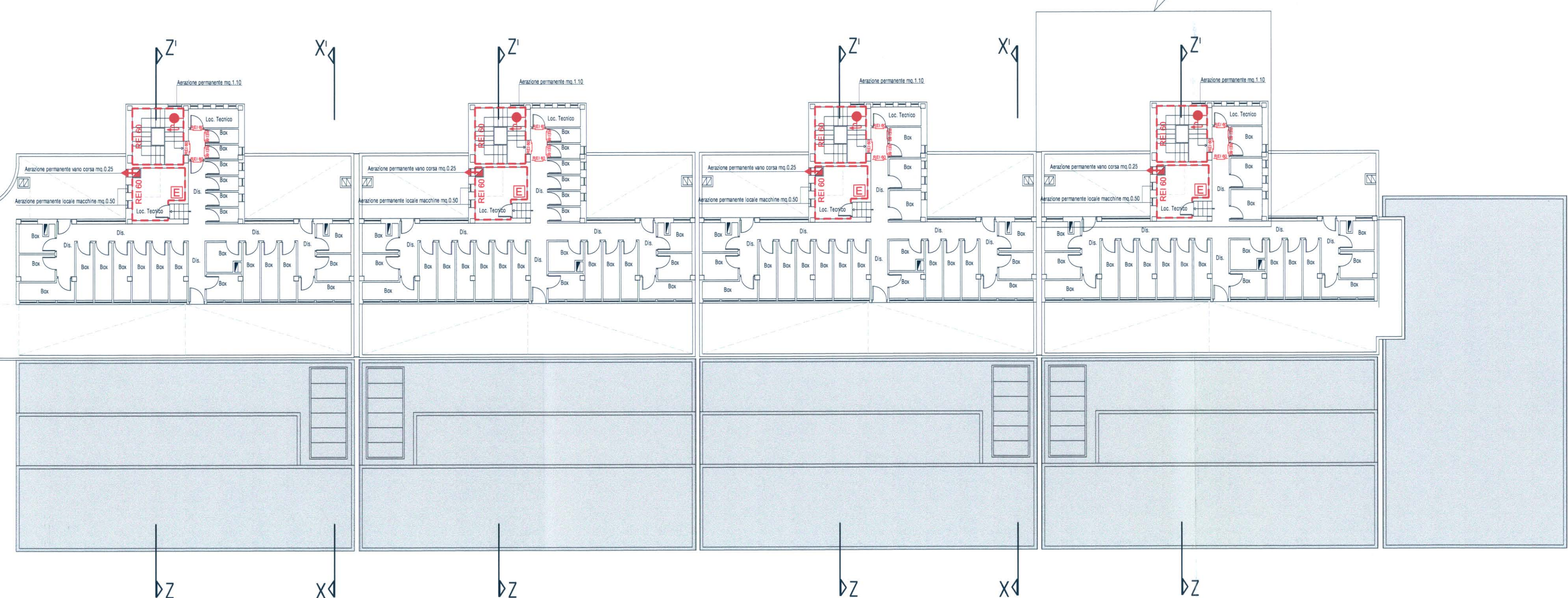
Piano Nono (accessori) scala 1:200
