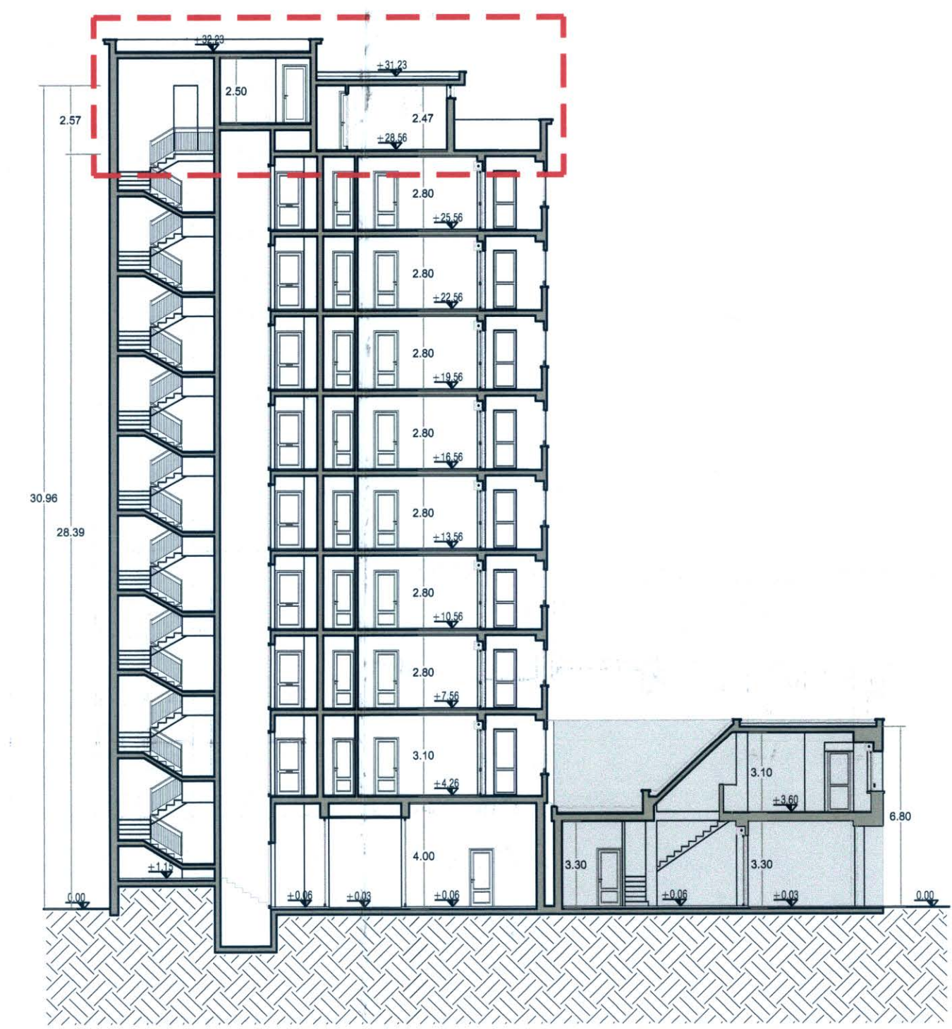
Sezione Z-Z' scala 1:200
