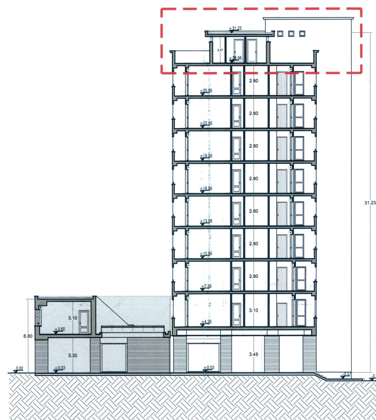
Sezione X-X' scala 1:200
