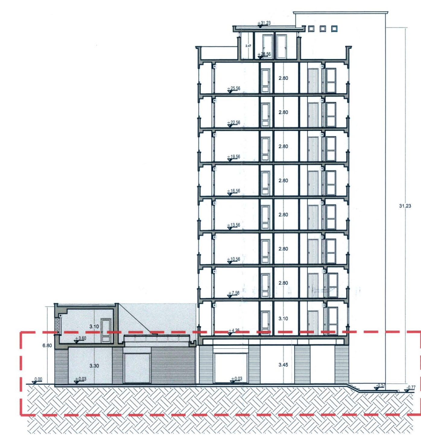
Sezione X-X' scala 1:200
