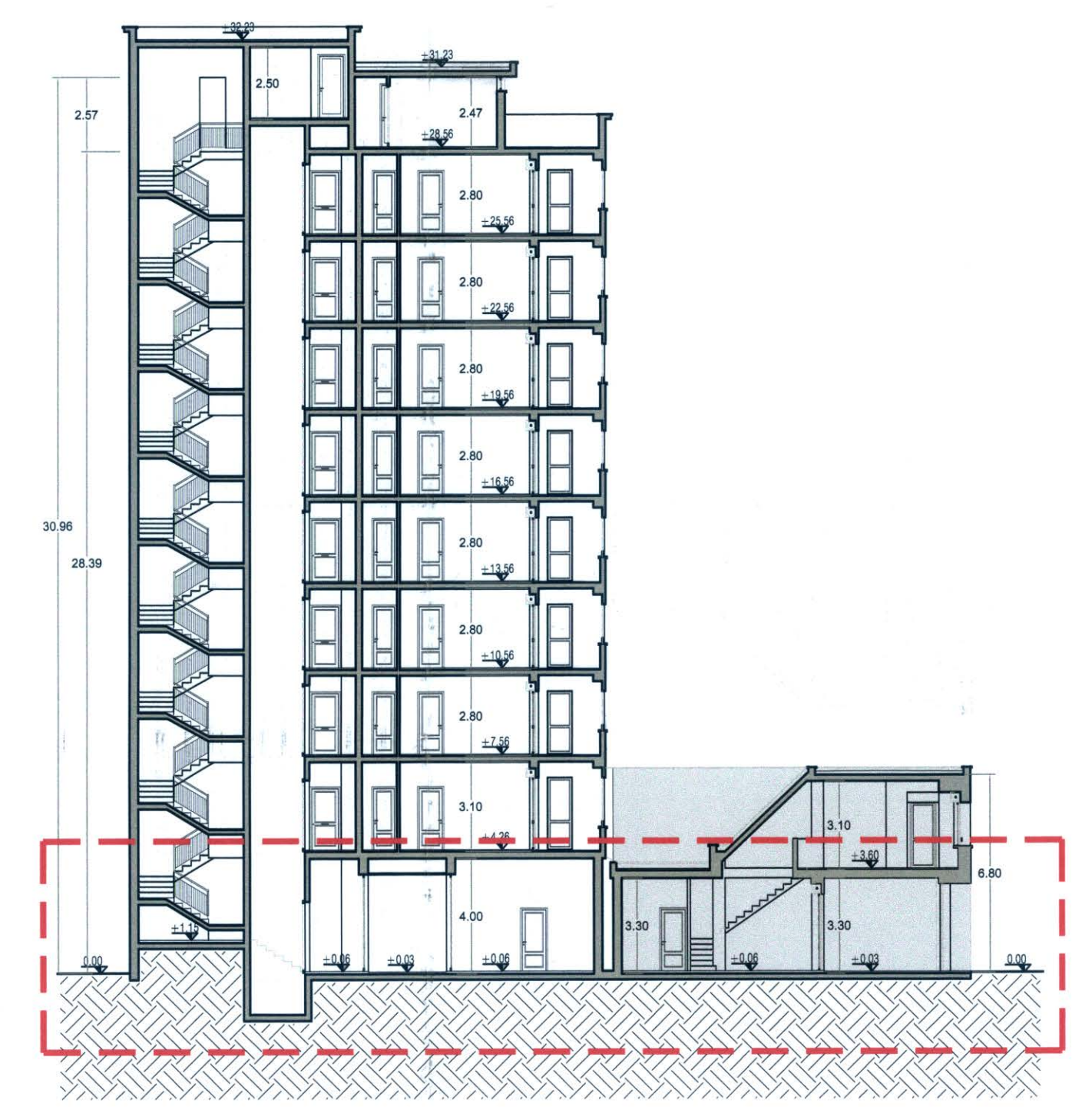
Sezione Z-Z' scala 1:200
