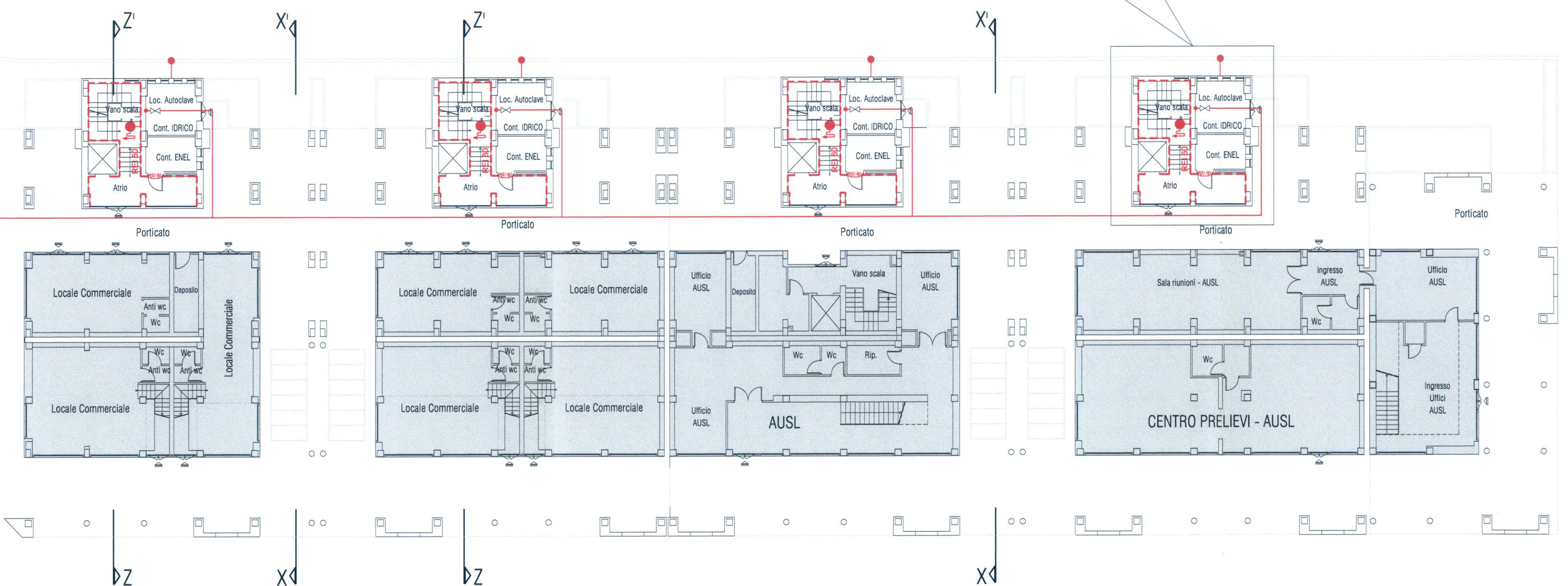
scala 1:200
